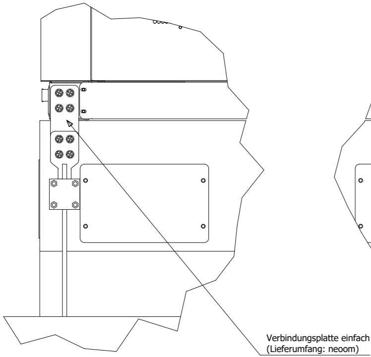
Erdungssanschlussplatte mit Kreuzverbinder und Verbindungsplatte einfach
