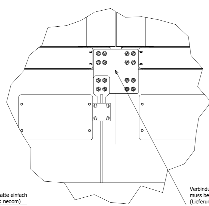
Erdungssanschlussplatte mit Kreuzverbinder und Verbindungsplatte doppelt
